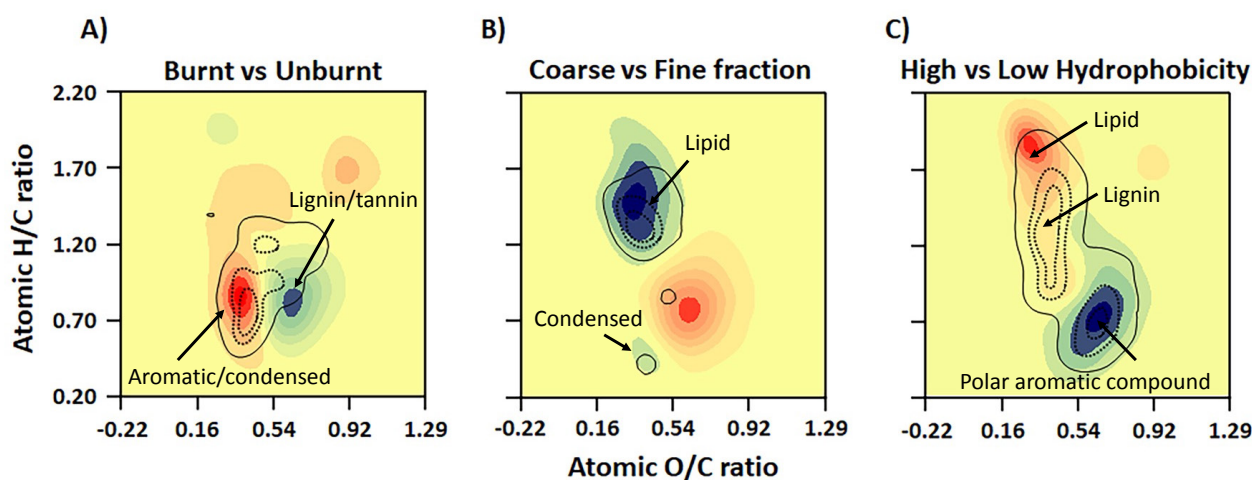
Figura 2 - Gráficos de densidad obtenidos a partir de los valores sustracción de las proporciones de las 1221 moléculas orgánicas comunes en muestras agrupadas en función de diferentes criterios: A) muestras afectadas por el fuego (rojo) frente a no afectadas (azul), B) fracciones gruesas (rojo) frente a fracciones finas (azul), y C) alta hidrofobicidad (rojo) frente a baja (azul). Los valores se representaron en el espacio definido por las relaciones atómicas H/C y O/C de los correspondientes compuestos (diagrama de Van Krevelen). Las diferencias más significativas entre los grupos de muestras se representan mediante un gráfico de contorno ( P < 0.1 en contorno externo, P < 0.01 en el interno).
