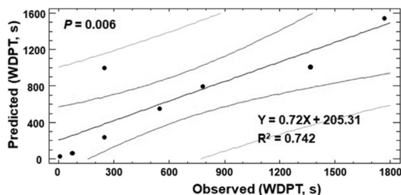
Figura 1 - Representación gráfica de la validación cruzada de valores observados frente a los predichos de la WDPT, obtenidos mediante el modelo de predicción para la WDPT generado por PLS ( R^2 = 0.742 ), utilizando 6 variables latentes sugeridas por los valores de error cuadrático medio (RMSE) y el criterio de información de Akaike (AIC).
