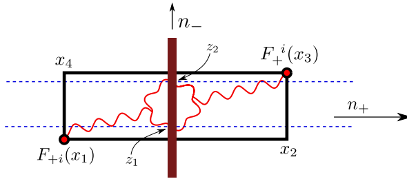
Fig. B.9. ImpactFactorNLO.
